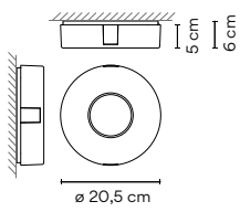
Surface Canopy S E1 Ø 205 mm. Watt-Optionen: <60W.
