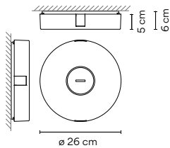
Surface Canopy M E2 Ø 260 mm. Watt-Optionen: >60W. <240W.
