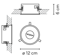
Built-in Canopy E3 Ø 120 mm. Watt-Optionen: >25W. <240W.
